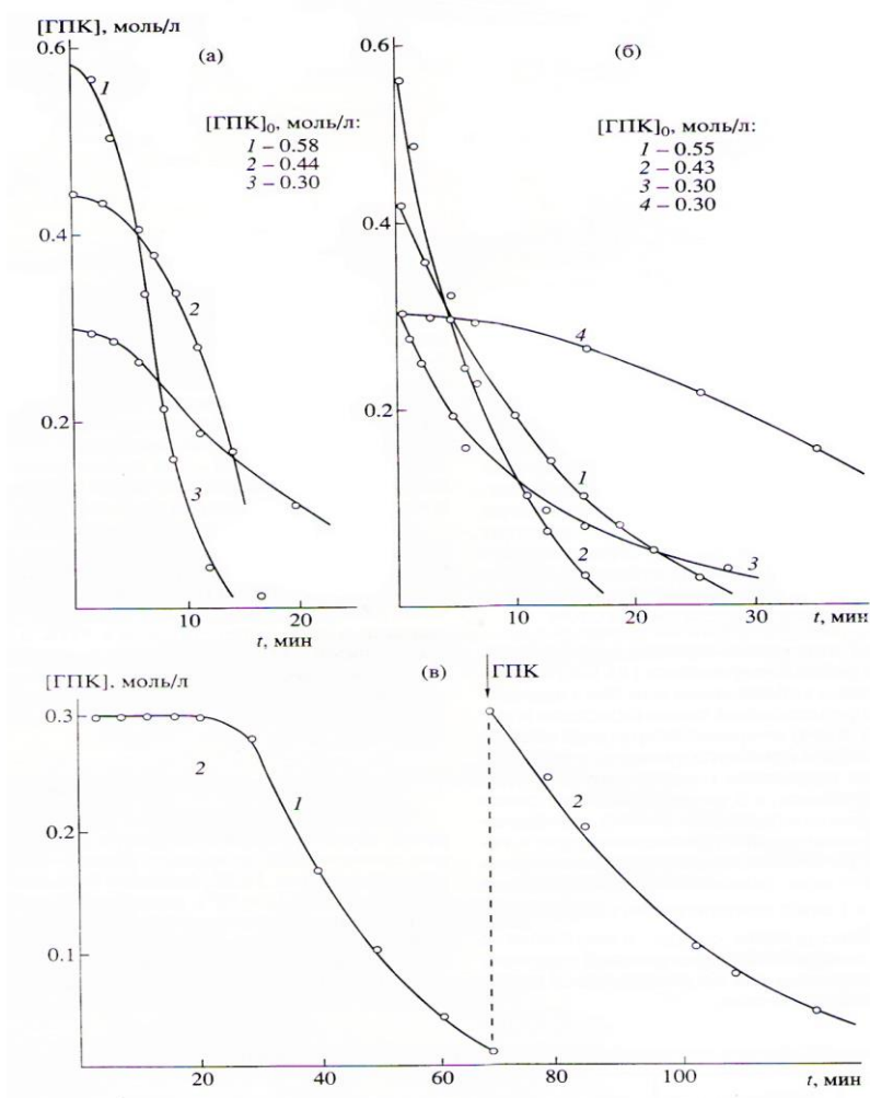
Рис. 1. Кривые расхождения ГПК с добавками ПФС і в атмосфере N 2 : а - 0.1 ммоль/л ПФС 2 , 110°C; б - 0.5 ммоль/л ПФС 1 , 100°C (1-3), 70°C (4); в - 0.3 ммоль/л ПФС 6 , 80°C (1) и после добавления свежей порции ГПК (2). Момент добавления ГПК показан стрелкой
